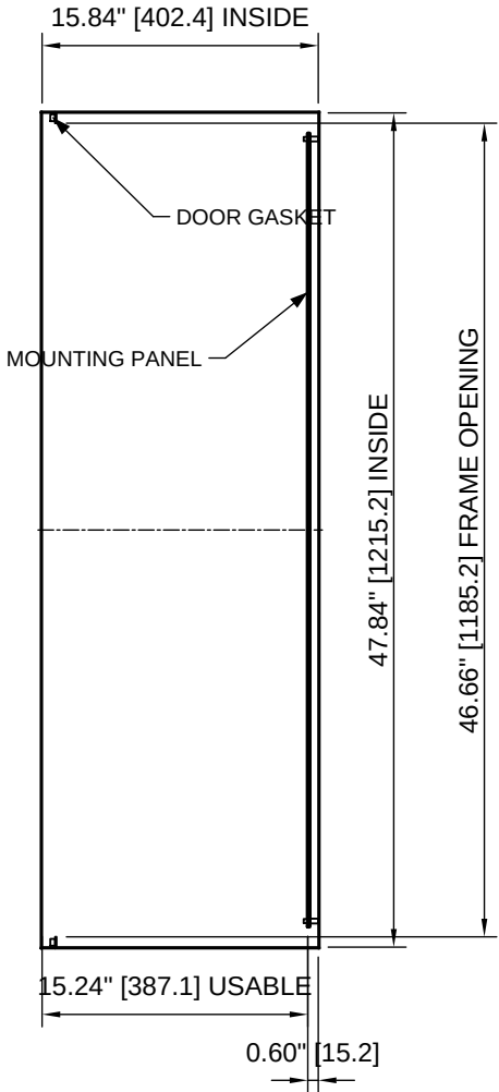
SECTION A-A INSIDE DIMENSIONS, DOOR LEFT
