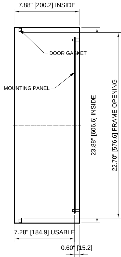
SECTION A-A INSIDE DIMENSIONS, DOOR LEFT
