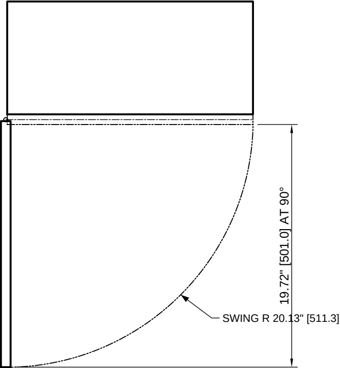
DOOR SWING (PLAN)
