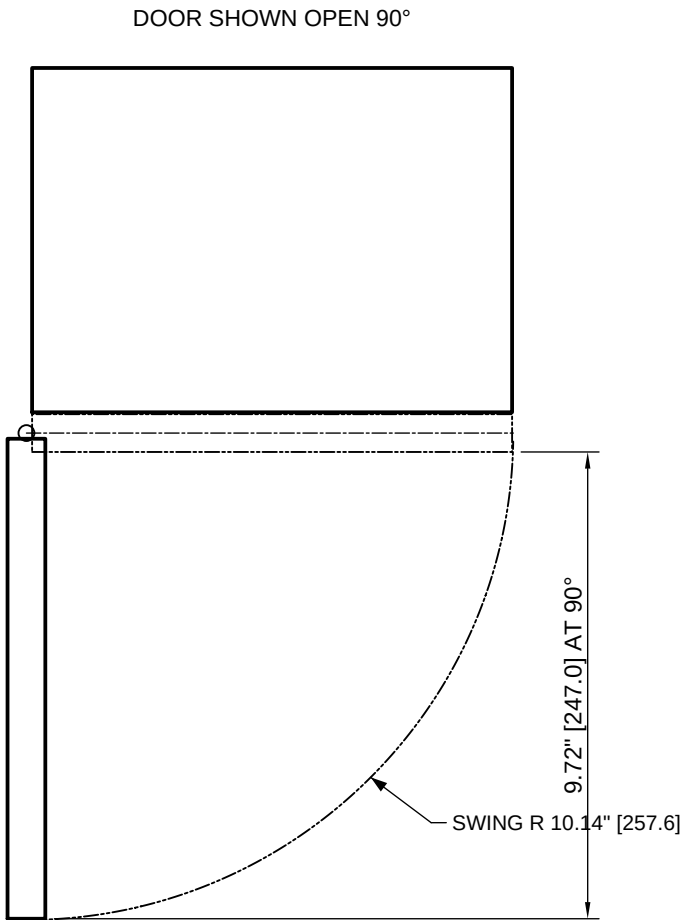
DOOR SWING (PLAN)
